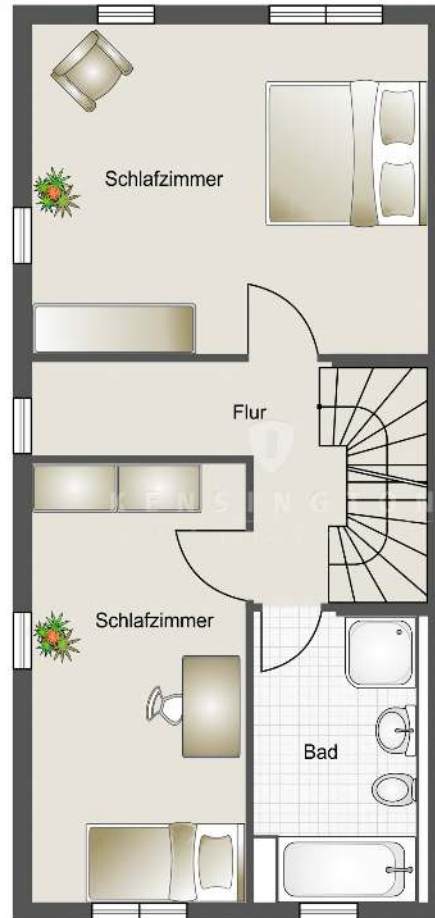
Obergeschoss
