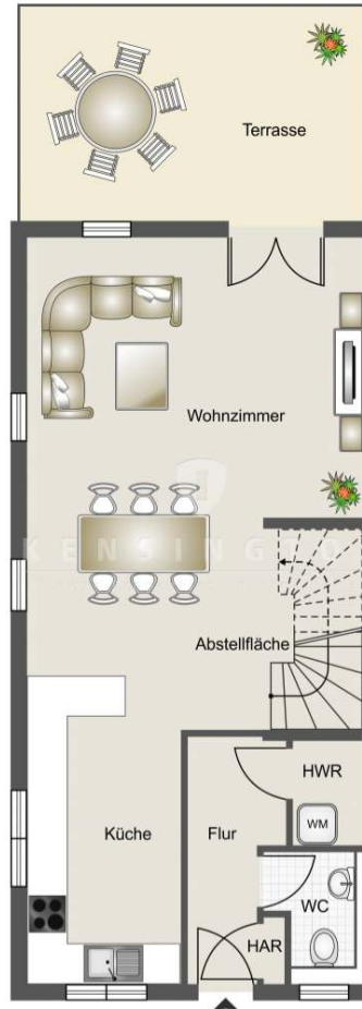
Erdgeschoss
