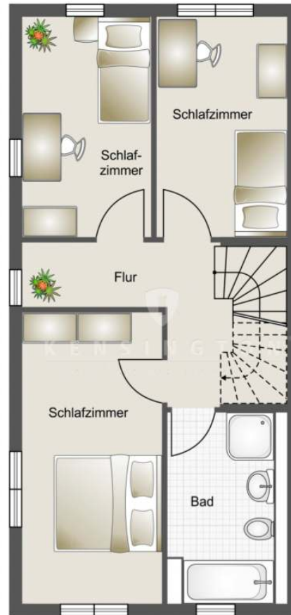
Obergeschoss
