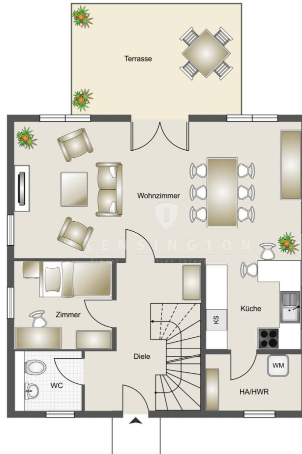
Erdgeschoss Variante
